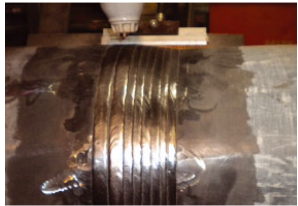
Instandgesetzte Welle
