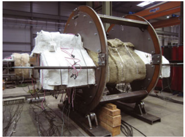
Erleichterung des Schweißprozesses am Rhönrad
