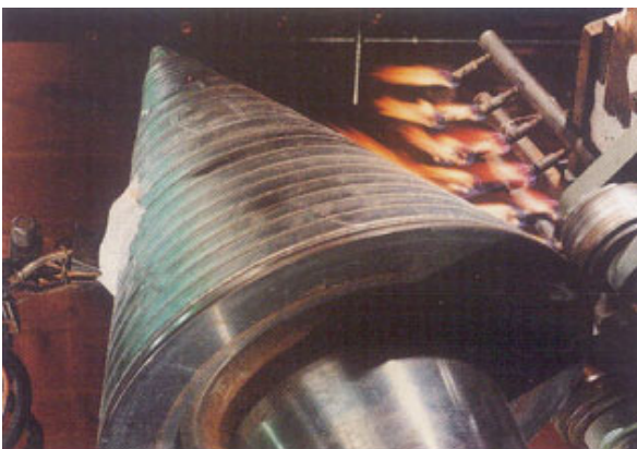
Axialwalze für Ringwalzwerk Werkstoff 56 Ni Cr Mo V
