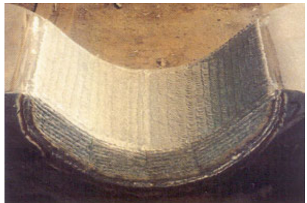
Schmiedesattel Werkstoff 56 Ni Cr Mo V
